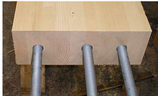
Abb. 7.2 Faserparallel eingeklebte Stahlstangen zur Übertra- gung planmäßiger Lasten
