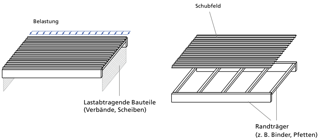
Abb. 3.2 Anordnung der Stahltrapezprofile parallel zu den Bindern und rechtwinklig zur Hallenlängsrichtung ohne zusätzliche Schubverbinder
