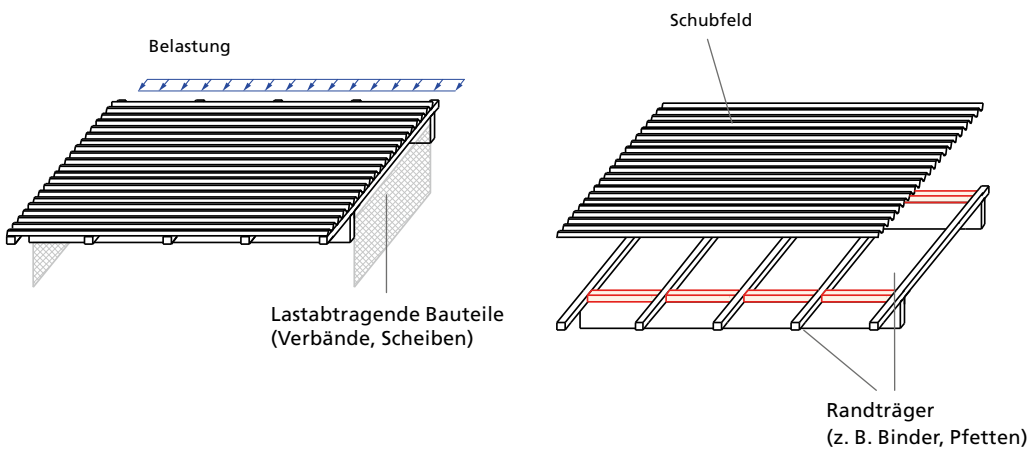
Abb. 3.3 Anordnung der Stahltrapezprofile parallel zu den Bindern und rechtwinklig zur Hallenlängsrichtung mit erforderlichen Schubverbindern
